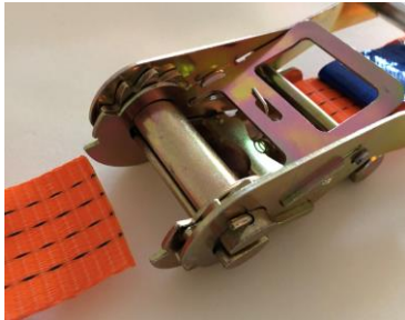
Åpen ende av båndet tres gjennom slissen foran på strammeren
