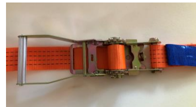
Når lasten skal frigjøres føres strammerens håndtak i 180° stilling. Strammeren er i fristilling og båndet kan trekkes ut.
