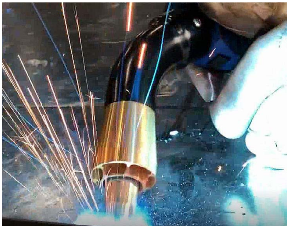
Høyvakuumpunktavsug gir bedre HMS og forbedret kvalitet. Foto: Reglo
